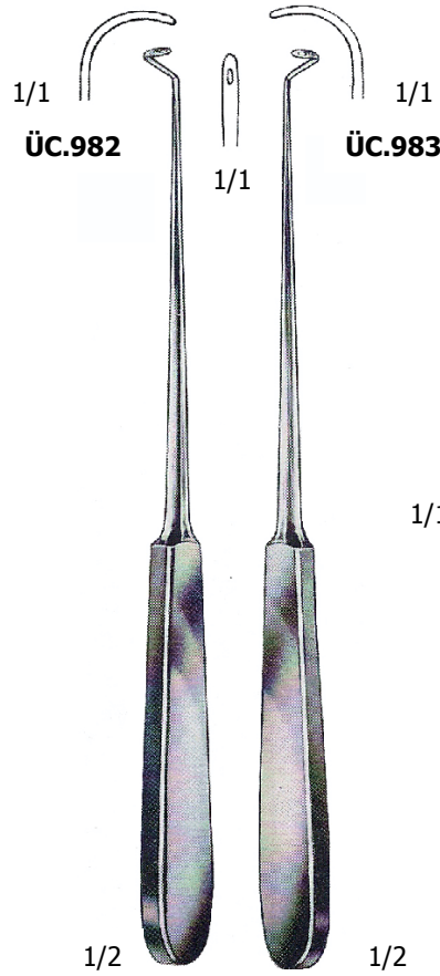
DESCHAMPS – 22.5 cm ÜC.982 Sağ/Right ÜC.983 Sol/Left Künt/Blunt
