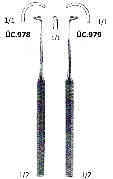
KRONECKER – 15.5 cm ÜC.978 Sağ/Right ÜC.979 Sol/Left Künt/Blunt
